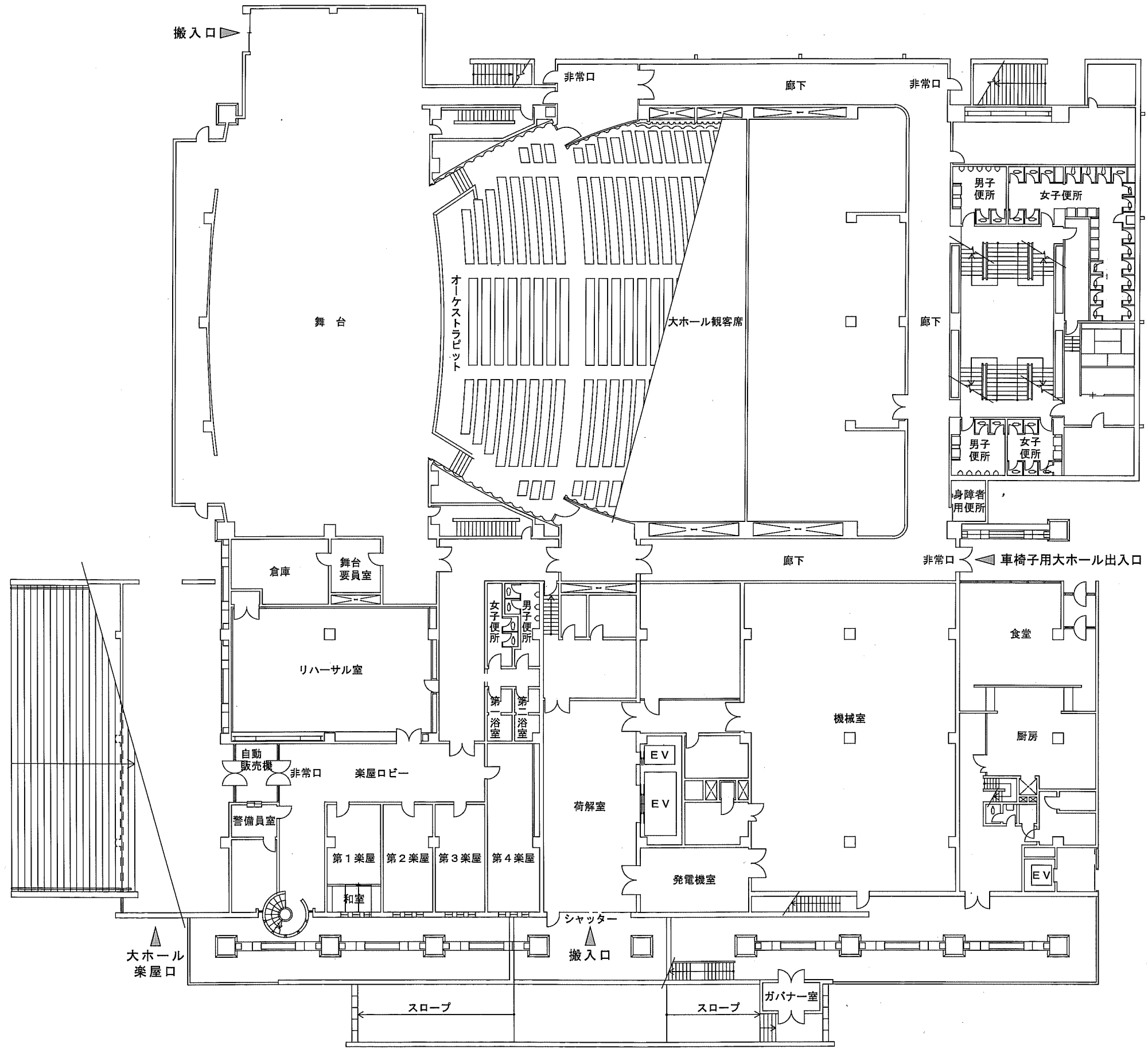
B 1 階平面図 S=1/300
