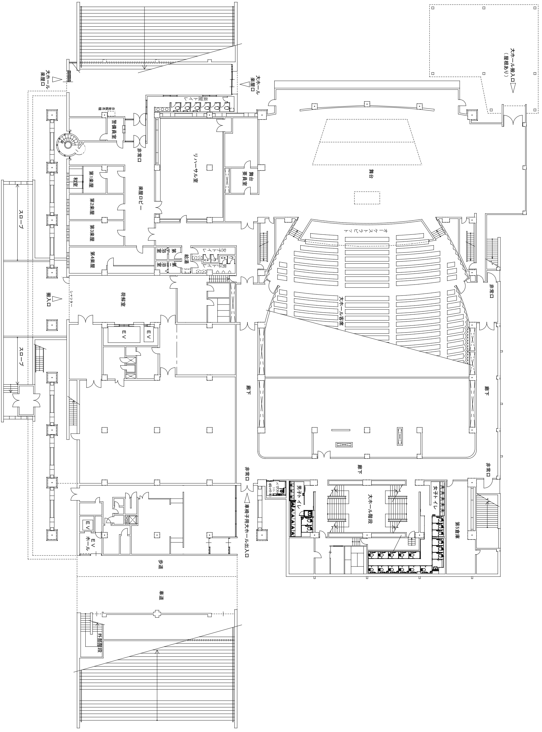
B 1 階平面図 A 3 : S = 1 / 3 0 0
